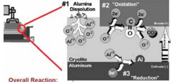
Şekil 2: Şematik olarak alüminyum elektrolizi
