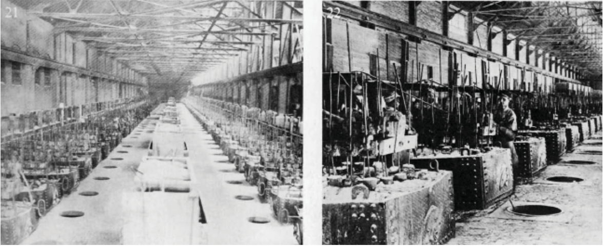
Şekil 3: Elektroliz hücreleri 1912 Alcoa
