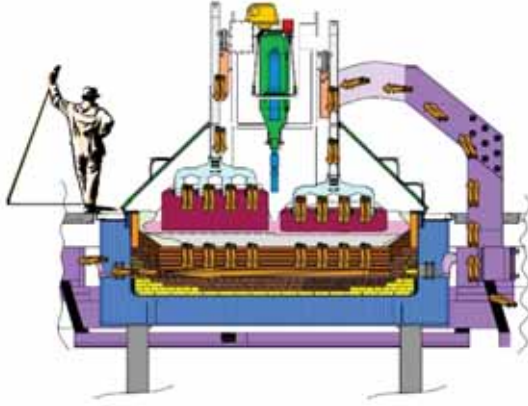
Şekil 10: Modern elektroliz hücresi
